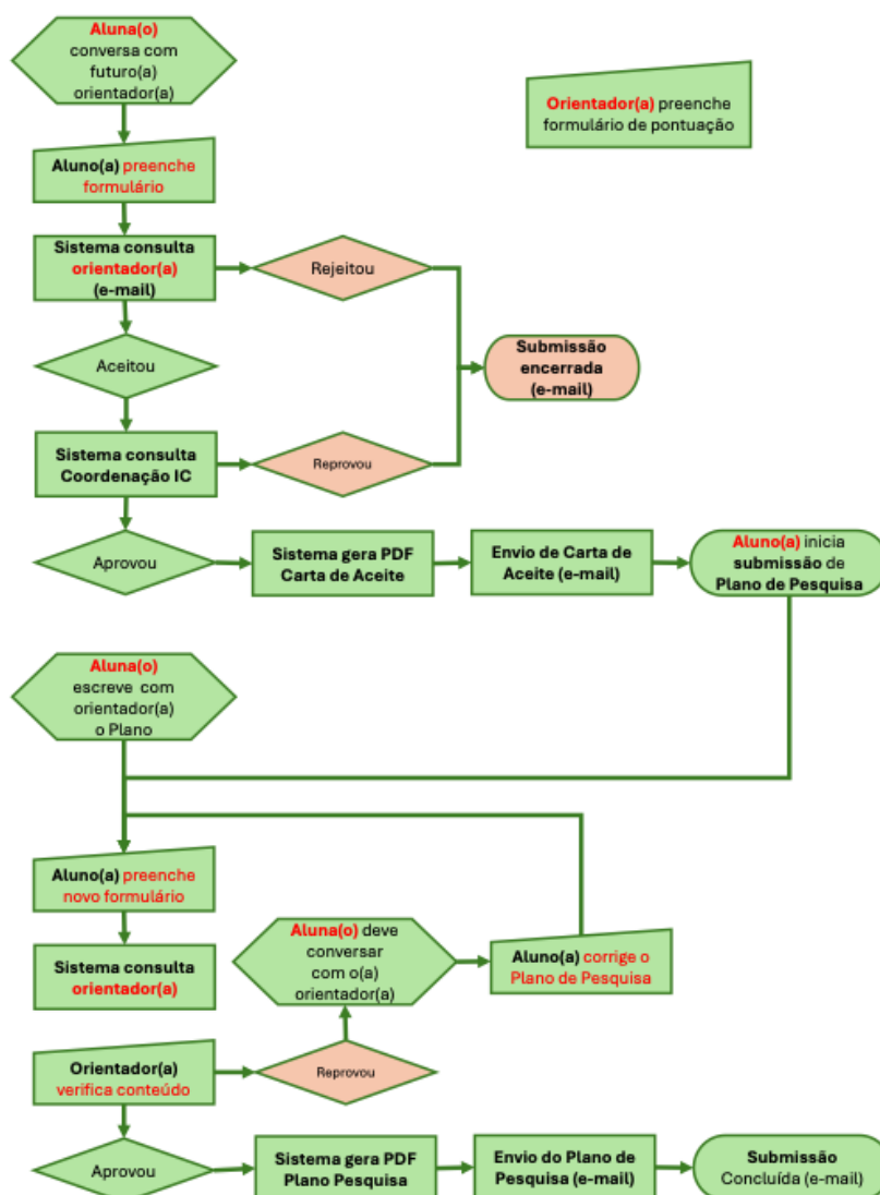
Figura 1. Fluxograma da submissão. Os prazos para preencher formulários e aceitar/rejeitar submissões estão na Tabela II. Falha no cumprimento dos prazos gera cancelamento da submissão.
