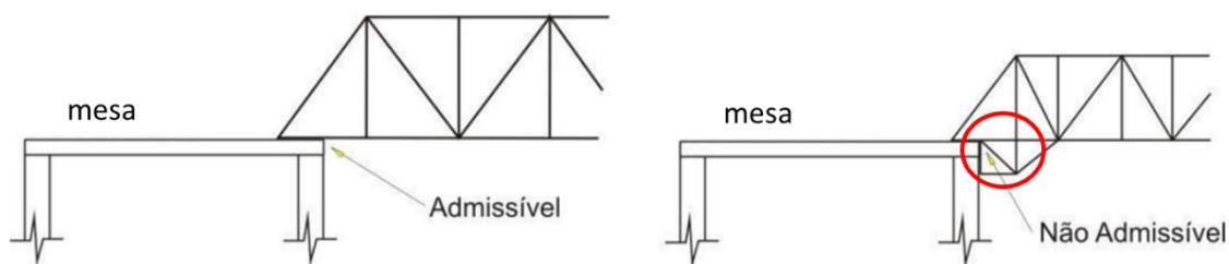
Figura 5 – Esquema de apoio da ponte
