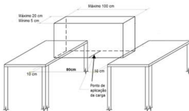
Figura 2 – Esquema da ponte
